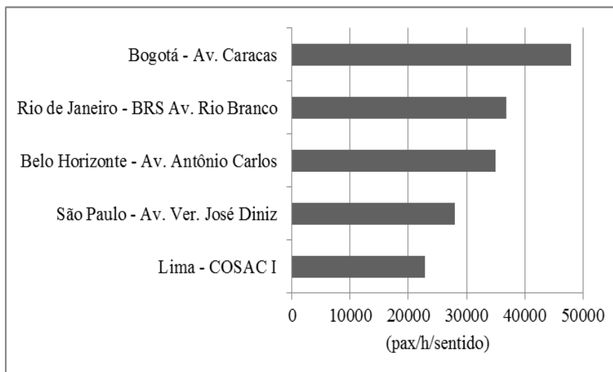
Figura 13: Demanda máxima na hora pico do trecho crítico no sentido mais carregado
