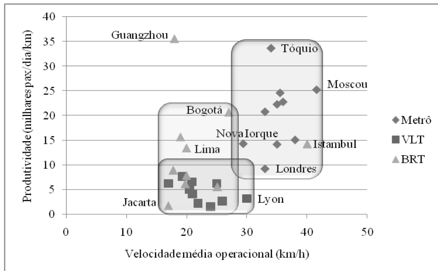
Figura 10: Produtividade de diferentes modais de transporte público urbano
