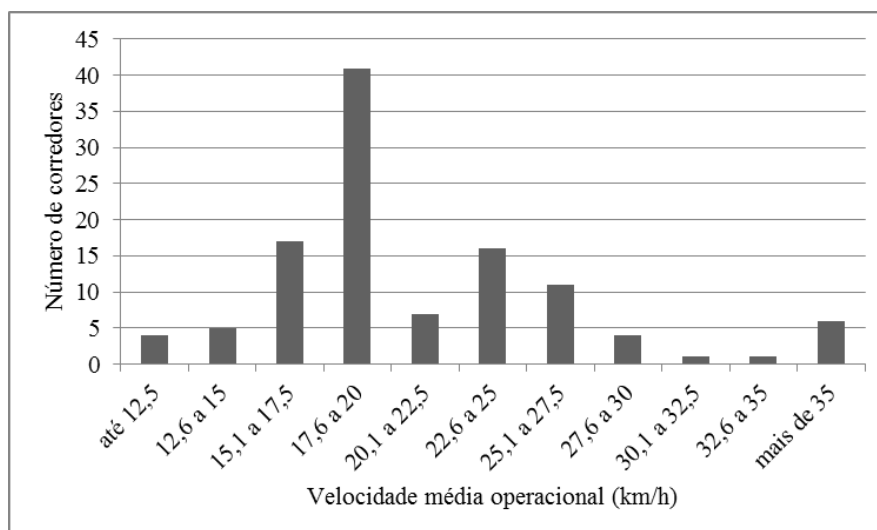
Figura 14: Distribuição dos corredores de acordo com a velocidade média operacional
