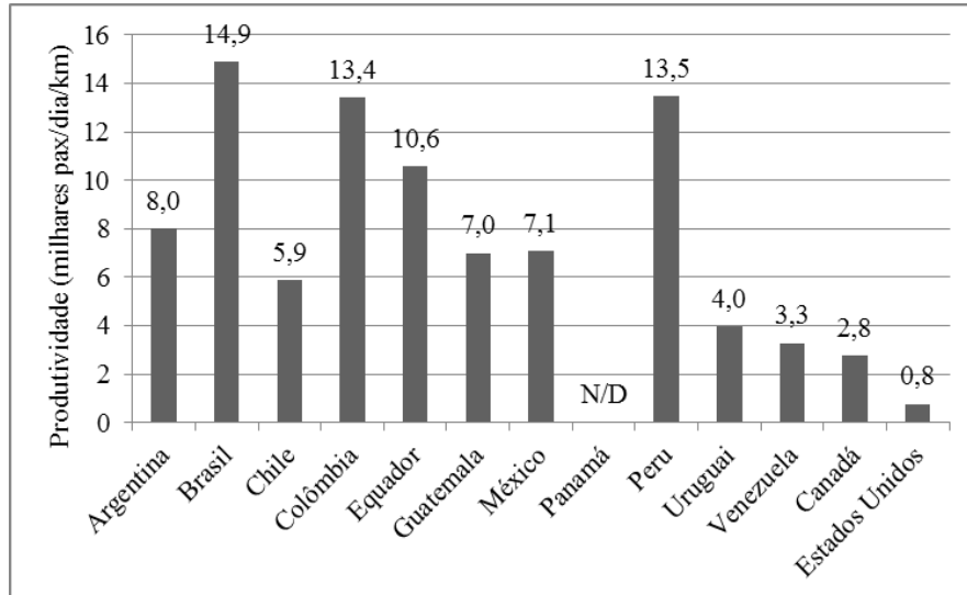
Figura 9: Produtividade dos corredores de ônibus e BRT por país
