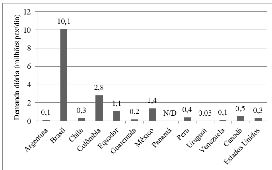
Figura 8: Distribuição da demanda em corredores de ônibus e BRT por país
